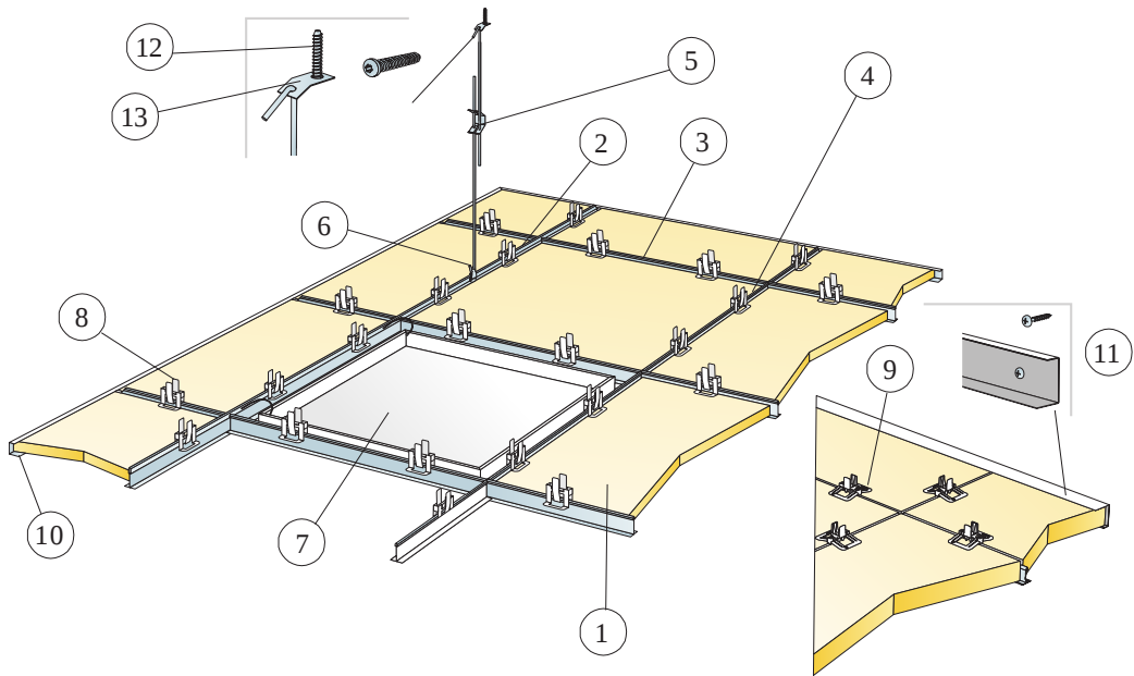
© Saint-Gobain Ecophon AB Schéma de montage (M395) pour Ecophon Hygiene Performance™ A C3
