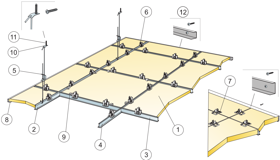
Schéma de montage (M266C4) pour Ecophon Hygiene Performance™ A C4
